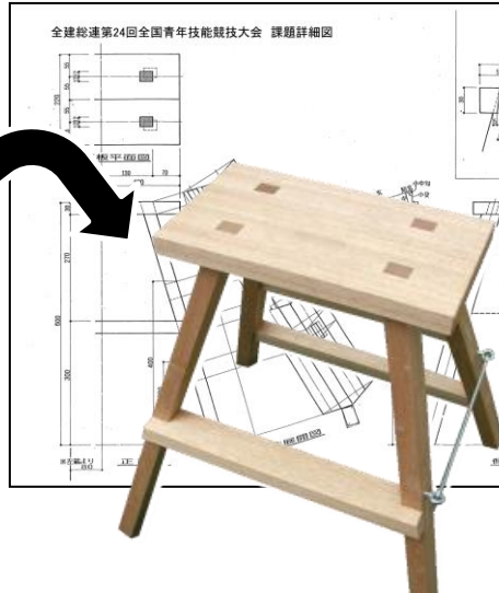
教材：四方転び踏み台
